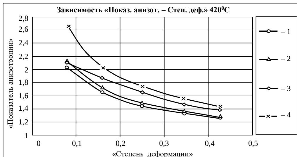
Рис. 2. Изменение показателя анизотропности ( \psi ) от степени поперечной деформации ( \varepsilon' ) при температуре 693 К и скоростях деформирования: 1 – при \dot{\gamma}_3 = 0,36 \cdot 10^{-3} \text{ м/с}^{-1} ; 2 – при \dot{\gamma}_4 = 0,15 \cdot 10^{-3} \text{ м/с}^{-1} ; 3 – при \dot{\gamma}_5 = 0,056 \cdot 10^{-3} \text{ м/с}^{-1} ; 4 – при \dot{\gamma}_6 = 0,023 \cdot 10^{-3} \text{ м/с}^{-1} .
