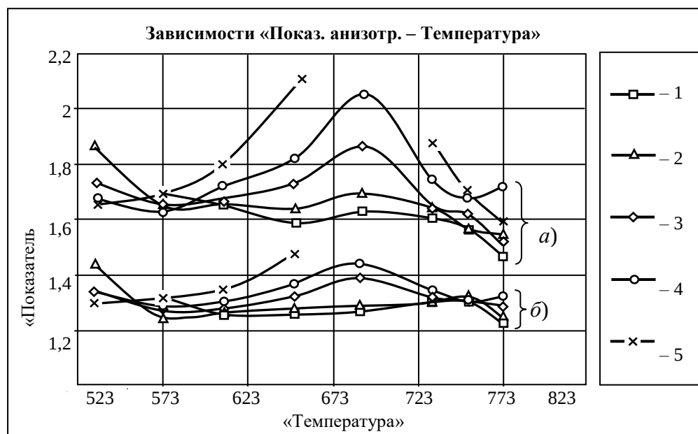
Рис. 4. Изменение показателя анизотропии от температуры ( \psi - T ) при скоростях деформирования: 1– \dot{\epsilon}_3 = 0,36 \cdot 10^{-3} \text{ м/с}^{-1} ; 2– \dot{\epsilon}_4 = 0,15 \cdot 10^{-3} \text{ м/с}^{-1} ; 3– \dot{\epsilon}_5 = 0,056 \cdot 10^{-3} \text{ м/с}^{-1} ; 4 – \dot{\epsilon}_6 = 0,023 \cdot 10^{-3} \text{ м/с}^{-1} ; 5 – \dot{\epsilon}_7 = 0,008 \cdot 10^{-3} \text{ м/с}^{-1} .
