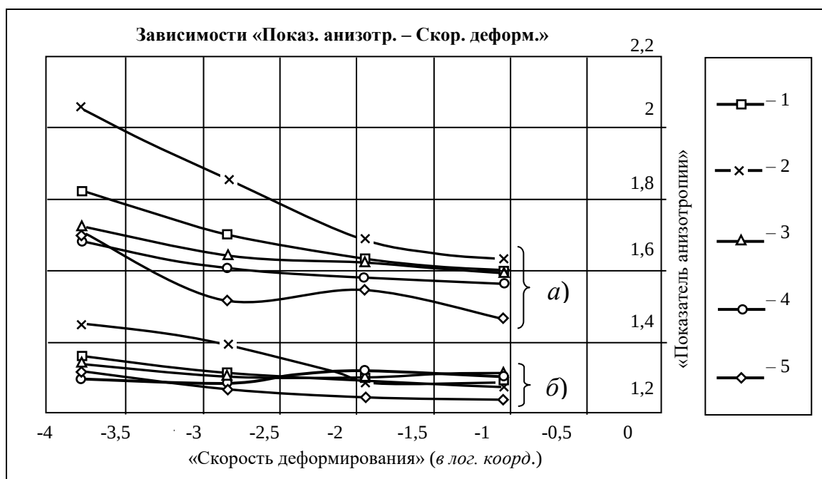
Рис. 3. Зависимости показателя анизотропности от скоростей деформирования ( \psi - \ln 9 ) при степенях деформации \epsilon' = 0,08333 - a ) и \epsilon' = 0,416667 - б ). Кривые 1...5 соответствуют температурным режимам: 1 – 653 К; 2 – 693 К; 3 – 733 К; 4 – 753 К; 5 – 773 К.
